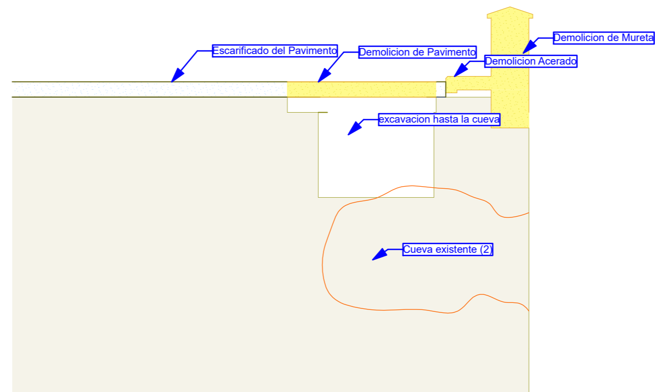
S-30 SECCION DEMOLICIONES 1:50
