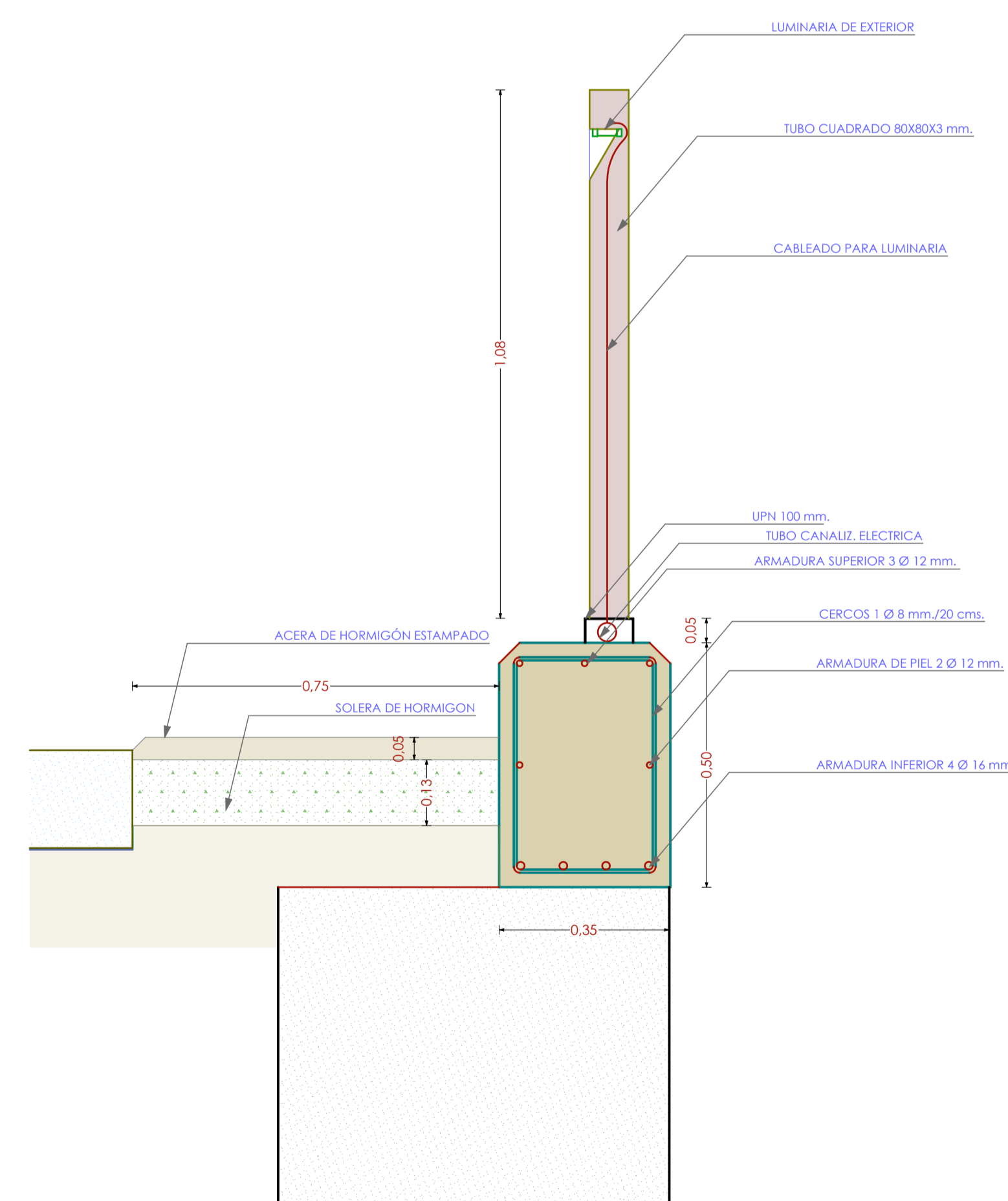
D-08 Detalle CONSTRUCTIVO 1:10
