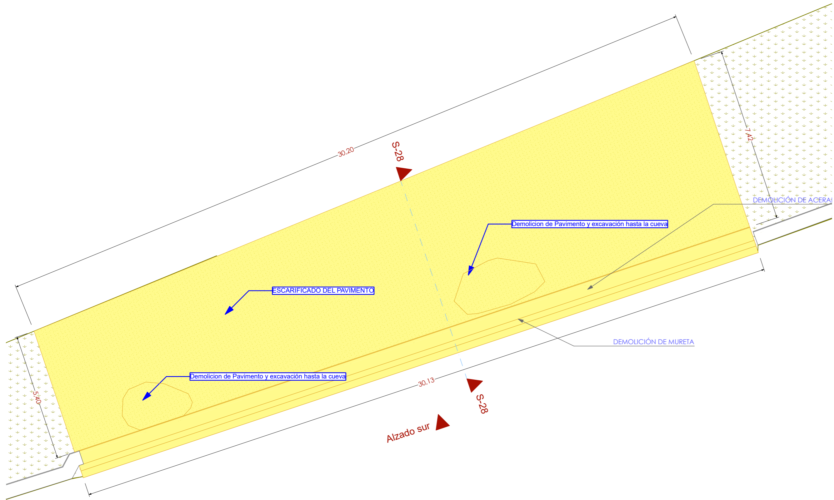
0. PLANTA DEMOLICIONES 1:100
