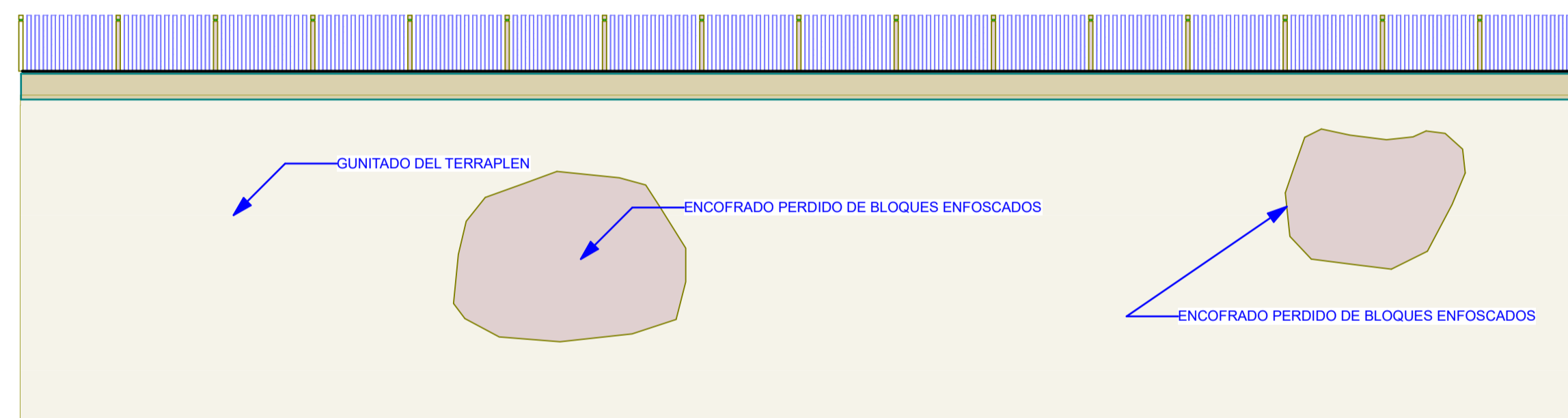
S-29 ALZADO DESDE EL BARRANCO 1:100
