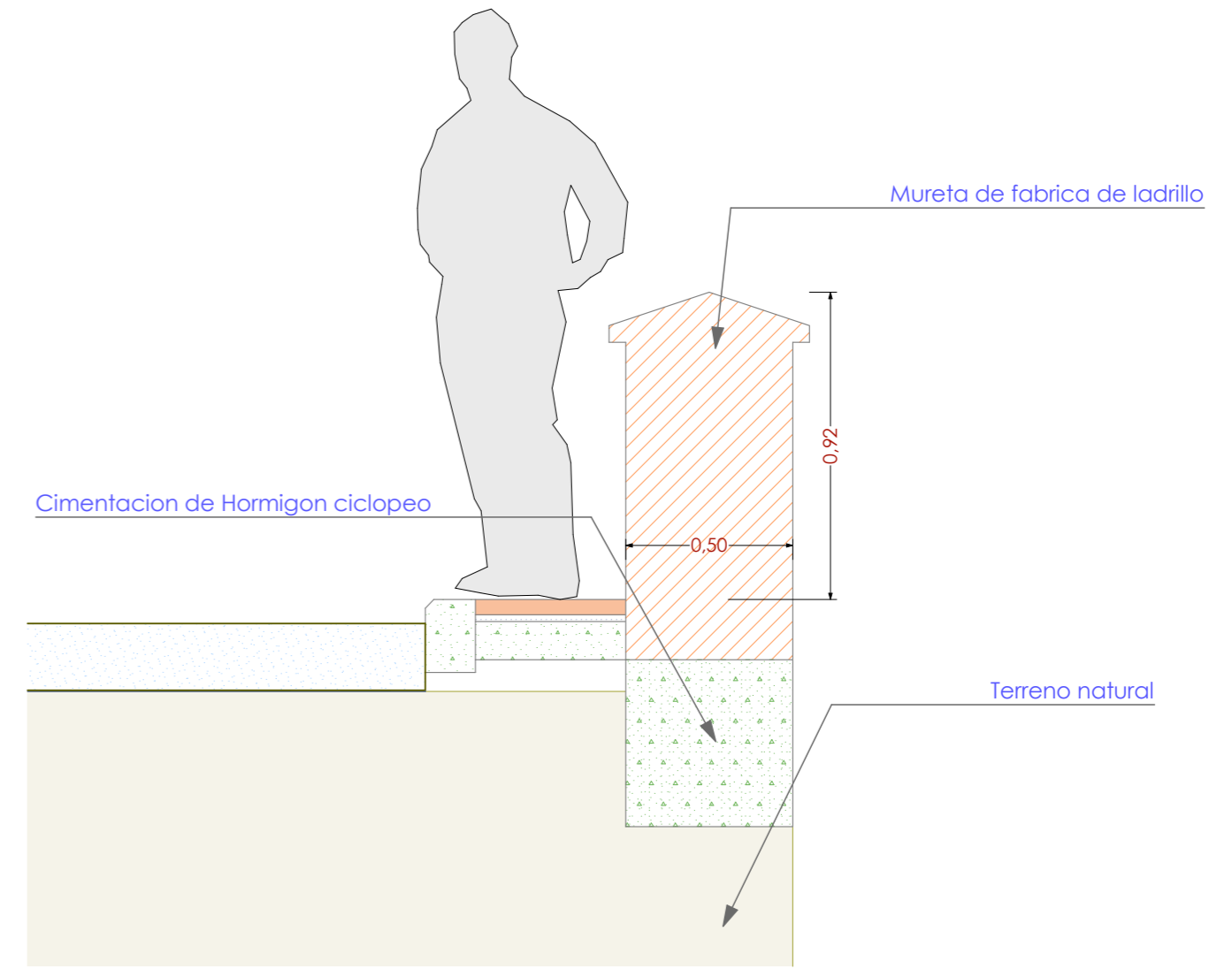
S-28 SECCION ESTADO ACTUAL 1:20
